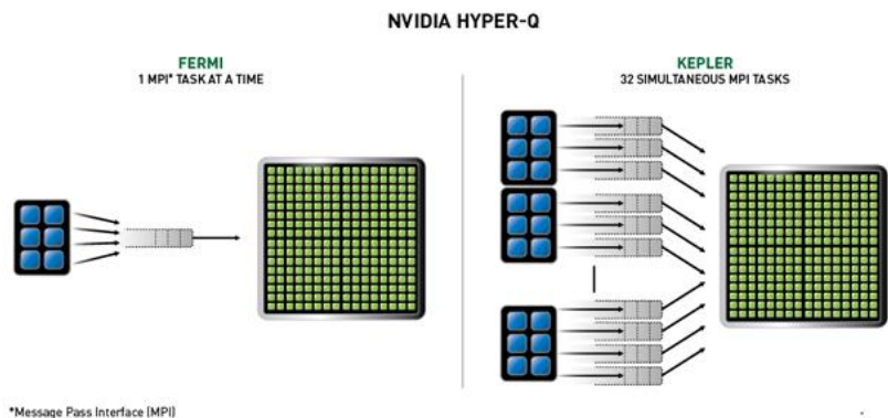
Рис. 3. Технология NVidia Hyper-Q
