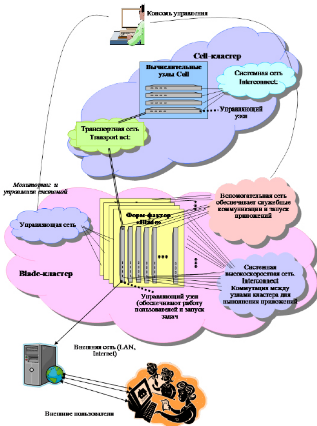
Рис. 2. Метакластерная гибридная архитектура опытного образца суперкомпьютера «СКИФ ОИПИ»
